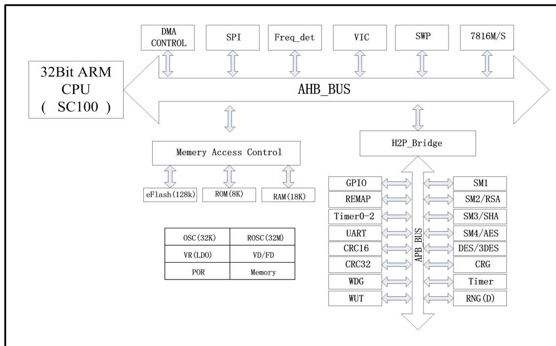
图 1 系统结构图
