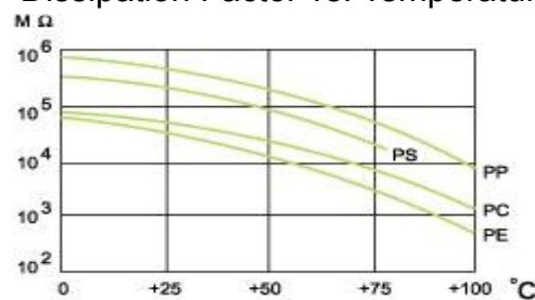
绝缘电阻与温度的关系
