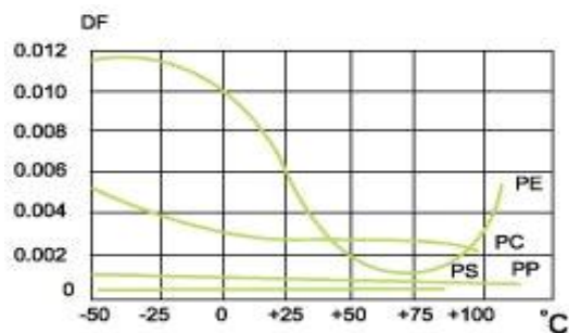
损耗角正切与温度的关系 Dissipation Factor vs. Temperature
