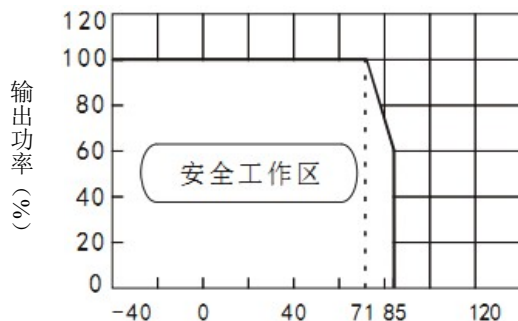
温度曲线图
