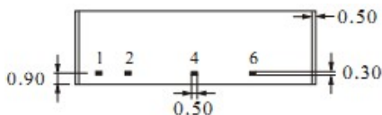
底视图
