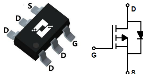
SOT23-6L
