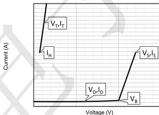
Fig.4 - VI Curve
