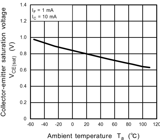
Fig. 11.9 V_{CE(sat)} - T_a
