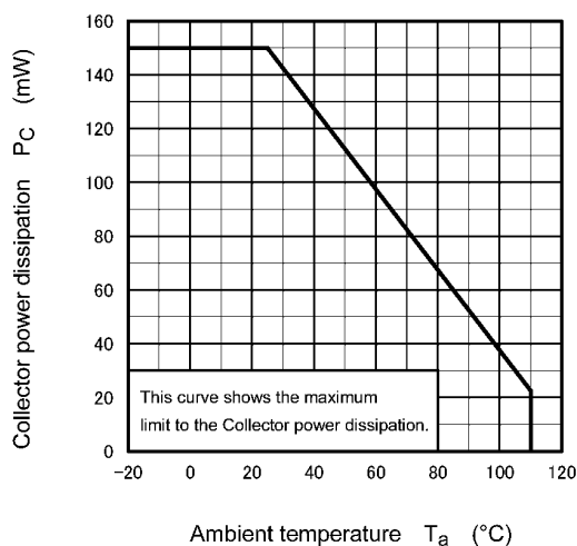
Fig. 11.2 P_C - T_a
