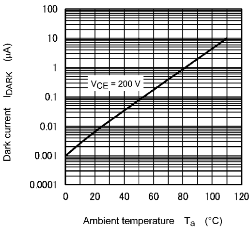
Fig. 11.8 I_{DARK} - T_a
