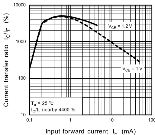
Fig. 11.11 I_C/I_F - I_F
