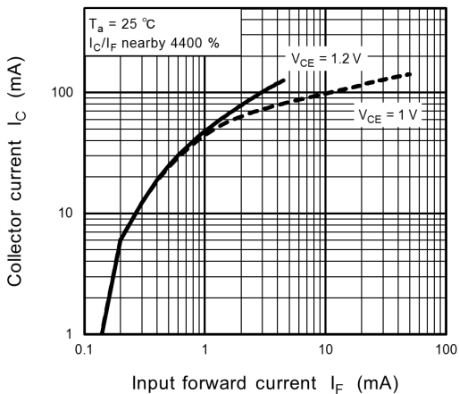
Fig. 11.10 I_C - I_F
