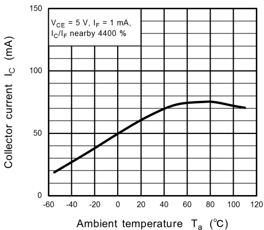
Fig. 11.12 I_C - T_a
