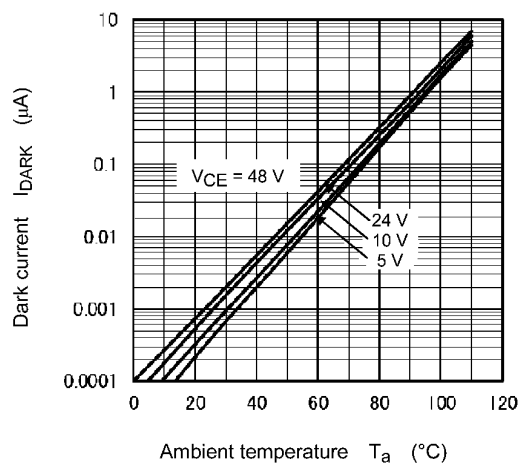
Fig. 11.10 I_{DARK} - T_a
