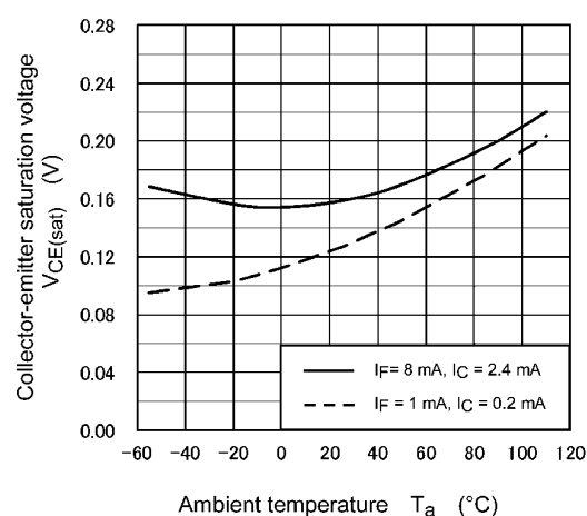
Fig. 11.12 V_{CE(sat)} - T_a
