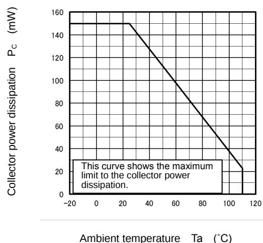
P_C - T_a
