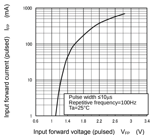
I_{FP} - V_{FP}
