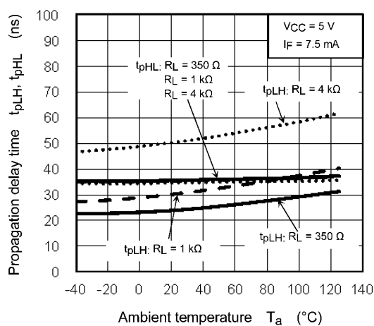
Fig. 13.2.11 t_{pLH} / t_{pHL} - T_a
