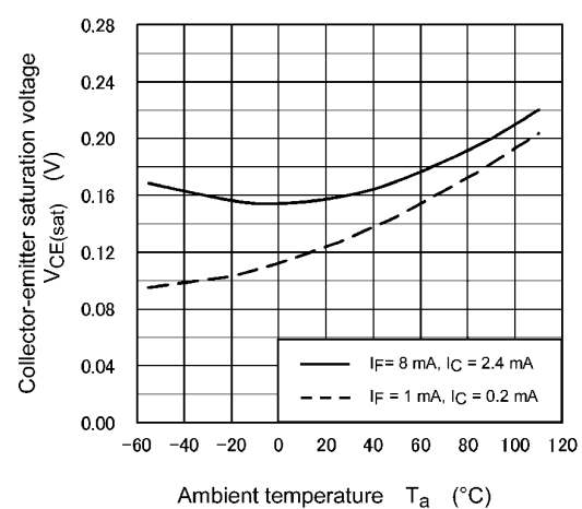
Fig. 11.12 V_{CE(sat)} - T_a
