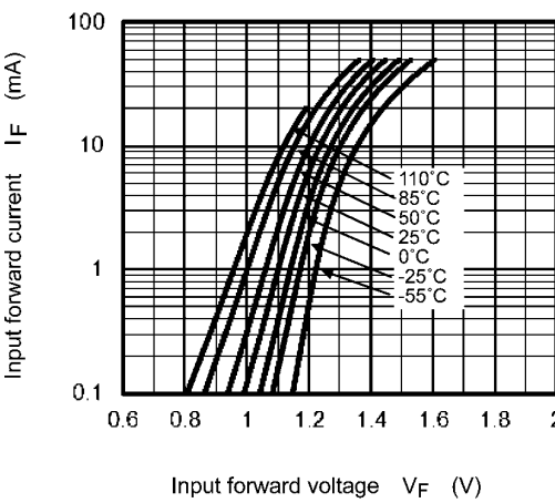
Fig. 11.4 I_F - V_F
