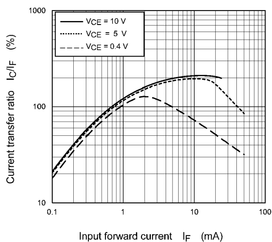
Fig. 11.11 I_C/I_F - I_F
