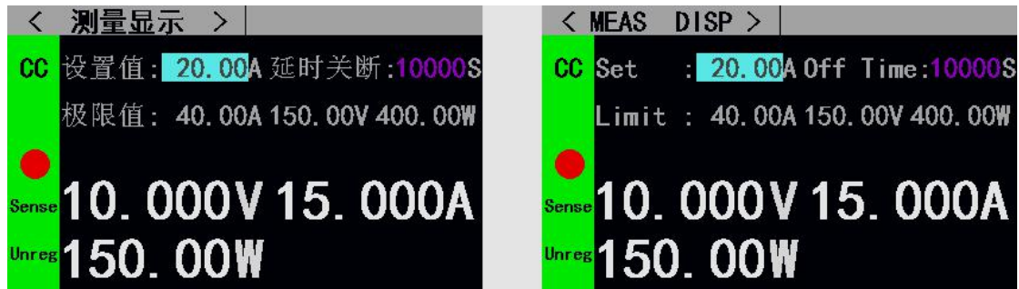
图 2.4.1 定电流测量模式
