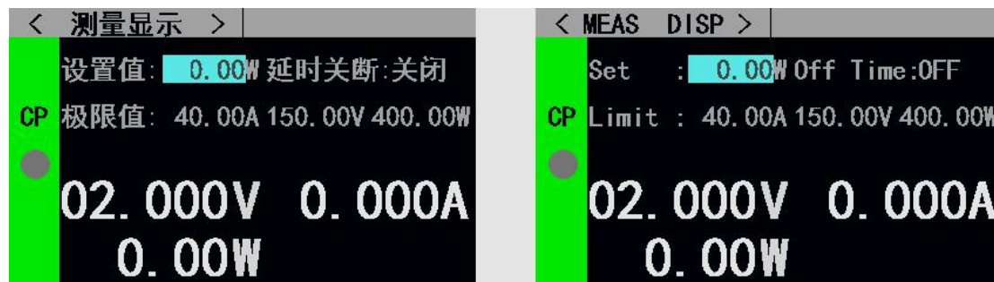
图 2.4.4 定功率测量模式
