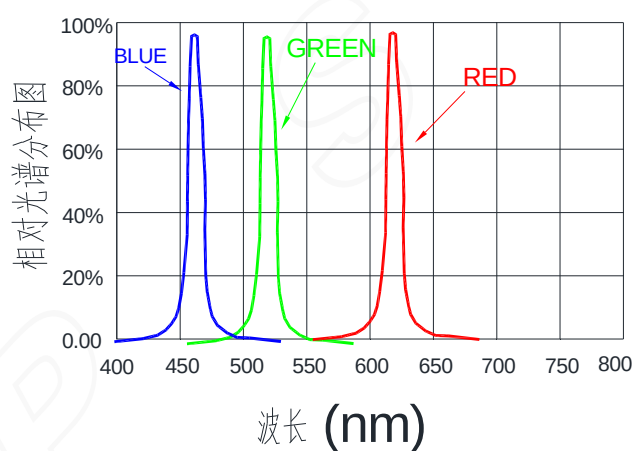
波长特性
