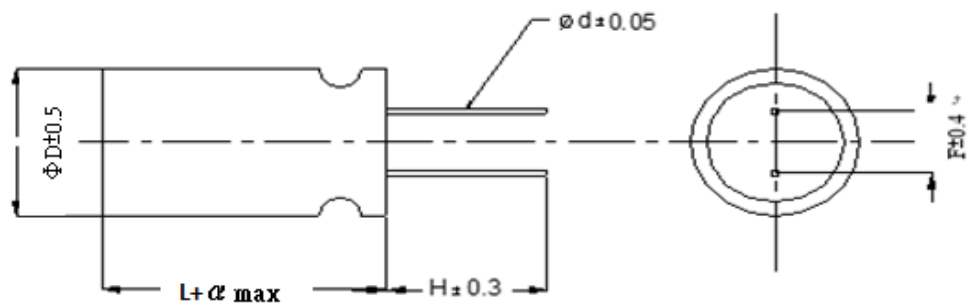
Fig. 2 Dimension
