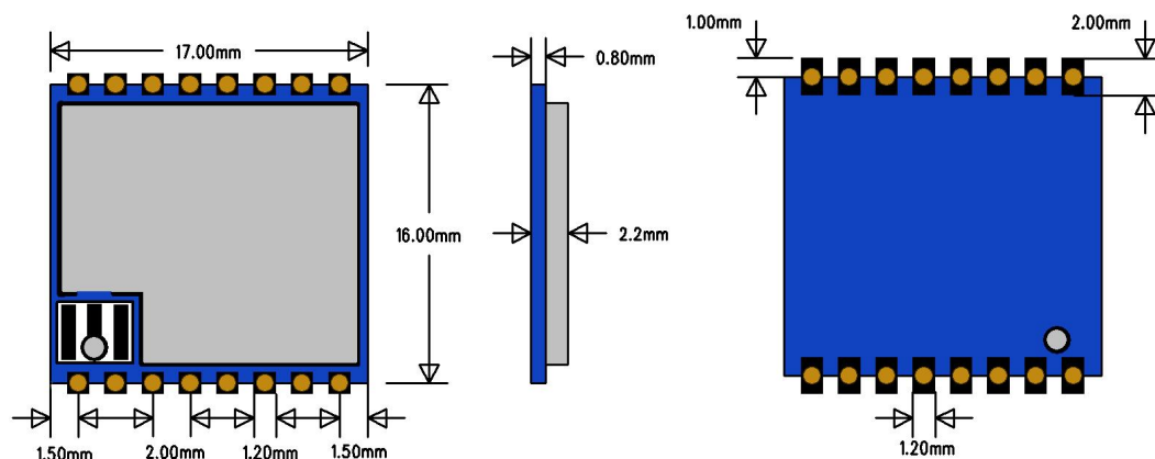
图 3. RC1262A 尺寸图
