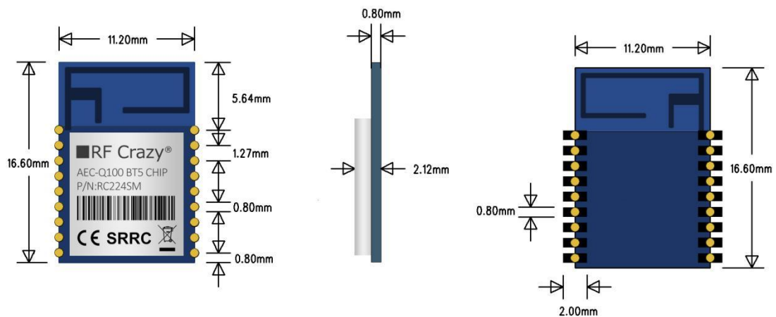
图 2. 模块尺寸图
