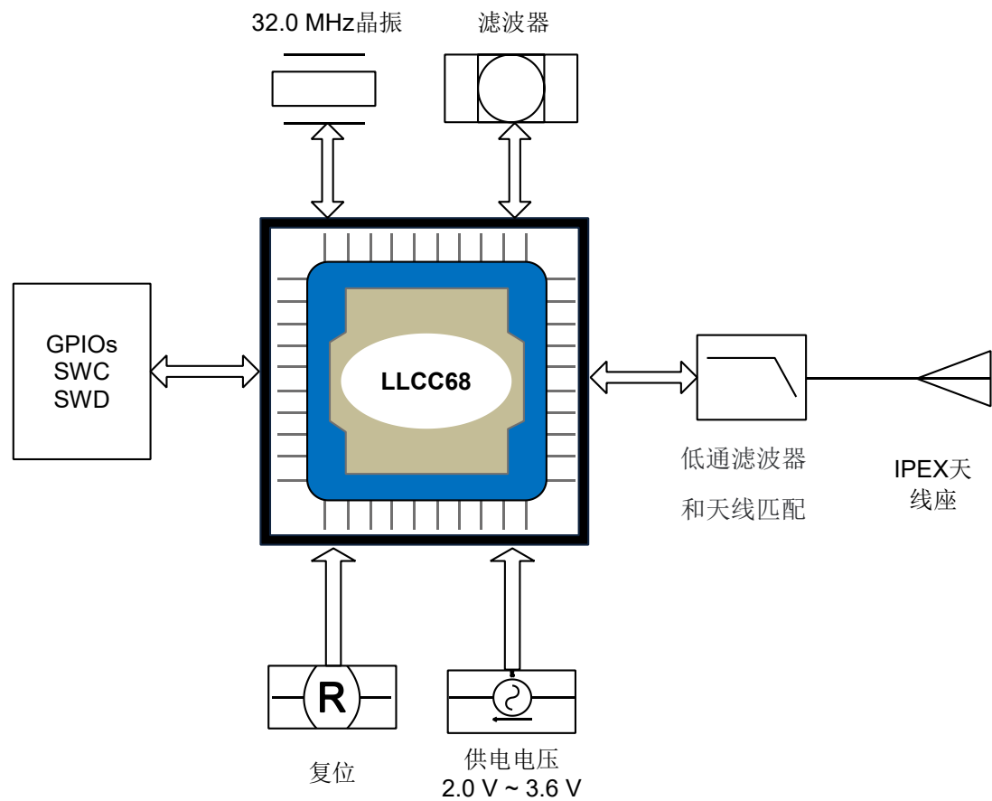
图 1. RC68A 设计框架图
