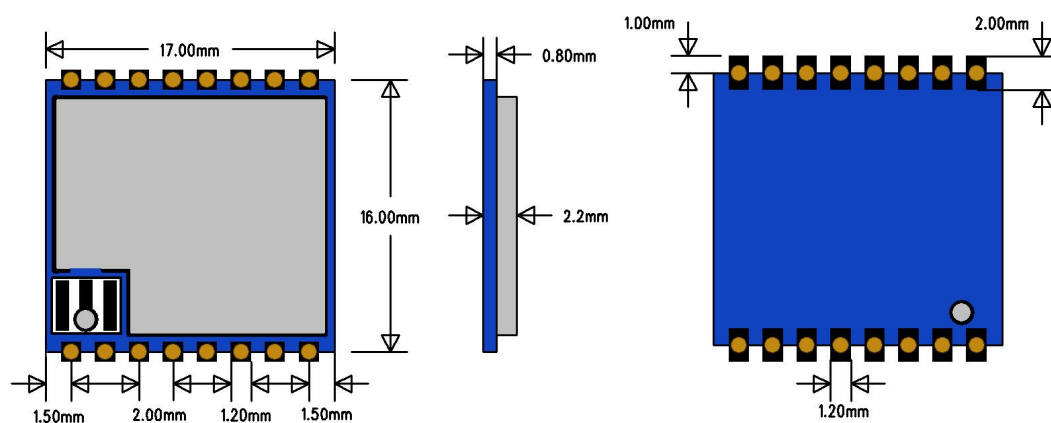
图 3. RC68A 尺寸图
