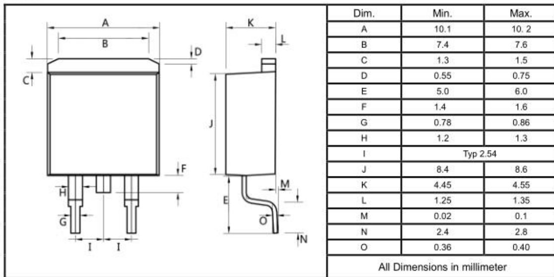
TO-263
