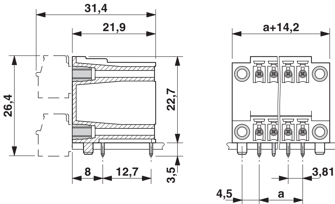
尺寸图
