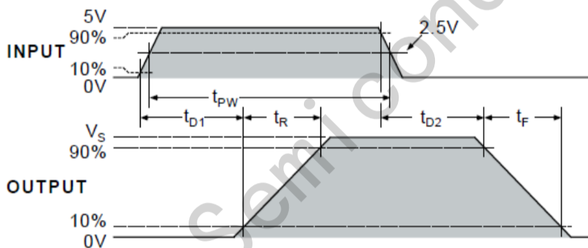
图 6-2 输入输出(B 通道同相)波形图
