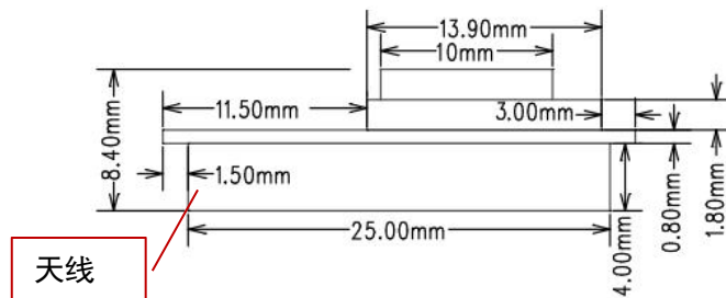
侧面视图
