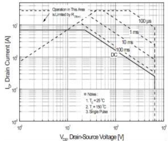
图 6-2 SIF7N65D(TO-220FP&220FJ)
