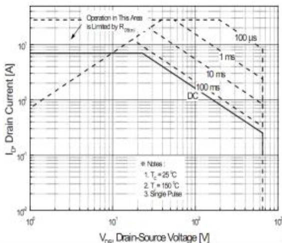
图 6-3 SIF7N65D(TO-262&263)
