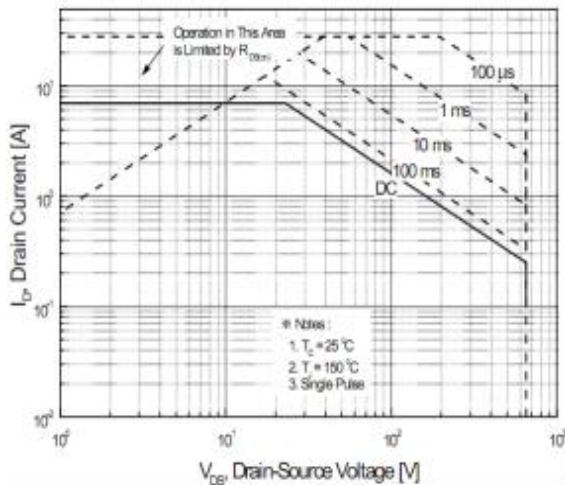
图 6-1 SIF7N65D(TO-220)
