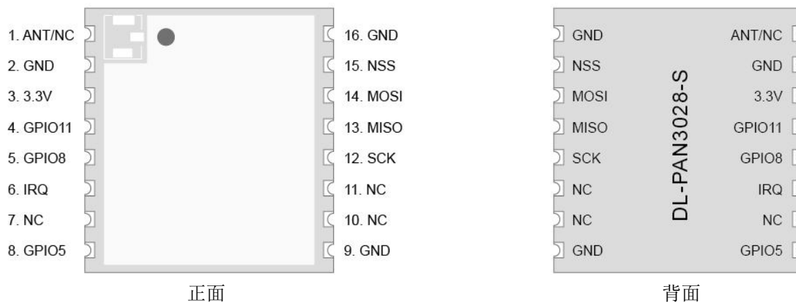
引脚示意图
