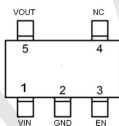
SOT-23-5
