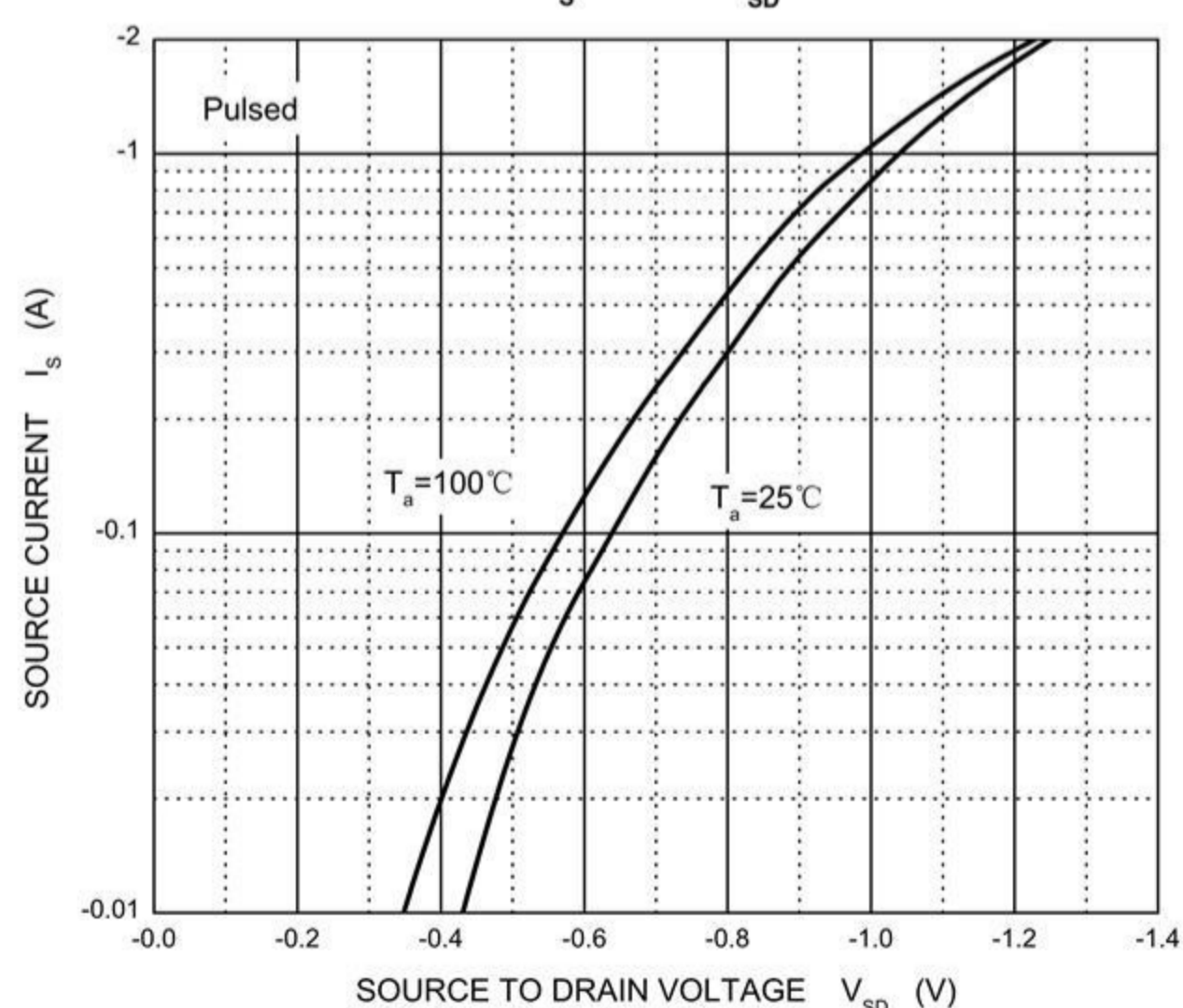
I_S — V_{SD}
