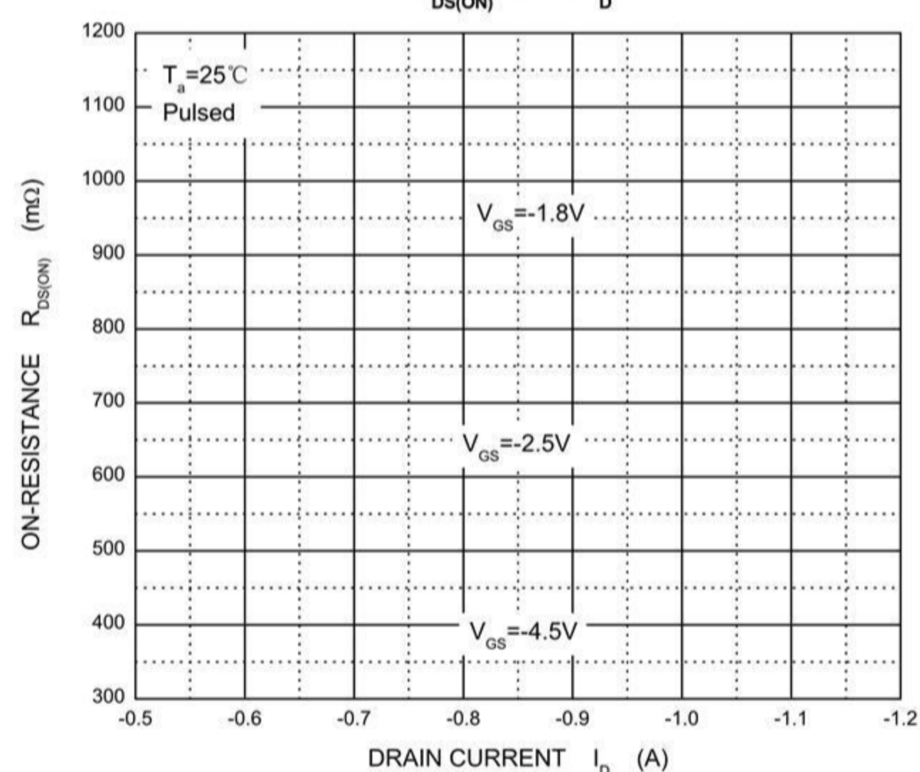
R_{DS(ON)} — I_D
