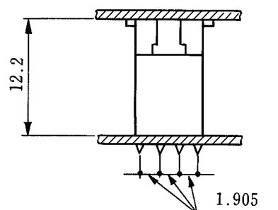
FX2C(A)-*P-1.27DSA(L)
