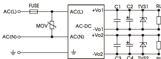
图 3. LHE15-20Dxx 系列
