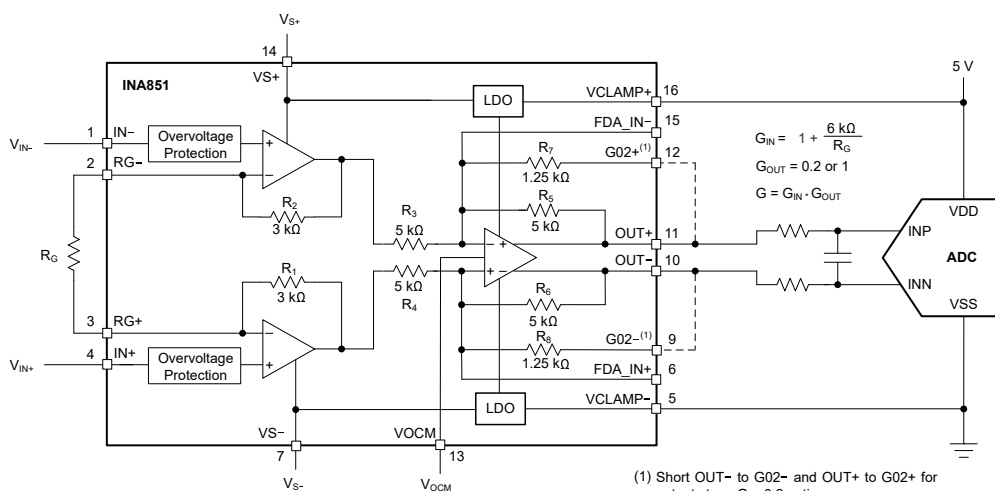
INA851 ADC 驱动器应用
