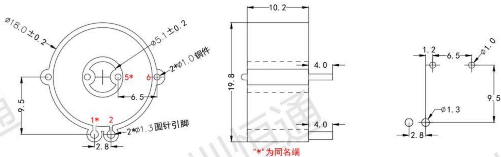
主视图
