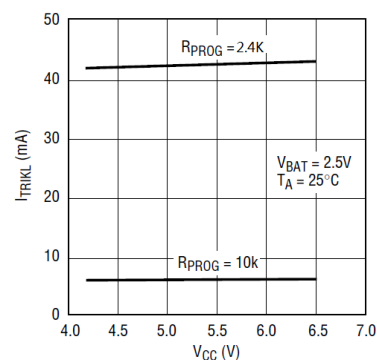
涓流充电电流 vs 电源电压
