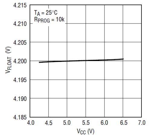
浮充电压 vs 电源电压
