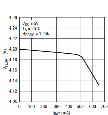
浮充电压 vs 充电电流
