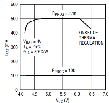
充电电流 vs 电源电压
