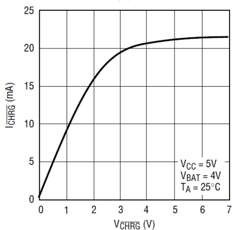
CHRG 引脚 I-V 曲线 (强下拉)
