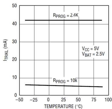
涓流充电电流 vs 温度
