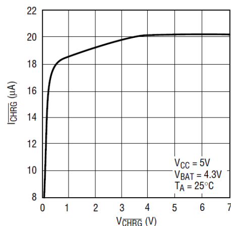
CHRG 引脚 I-V 曲线 (弱下拉)
