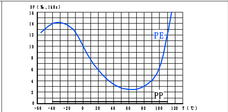
损耗角正切与温度的关系 Dissipation Factor vs. Temperature
