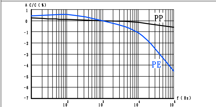
容量变化率与频率的关系 Capacitance vs. Frequency
