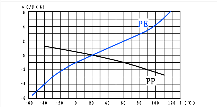
容量变化率与温度的关系 Capacitance vs. Temperature
