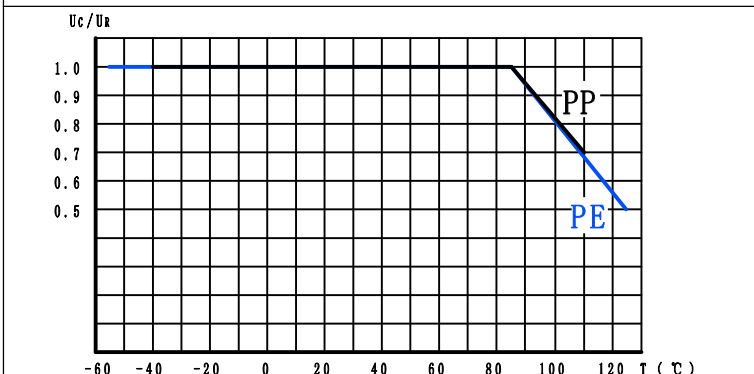
使用电压与温度的关系 Operation voltage vs. Temperature
