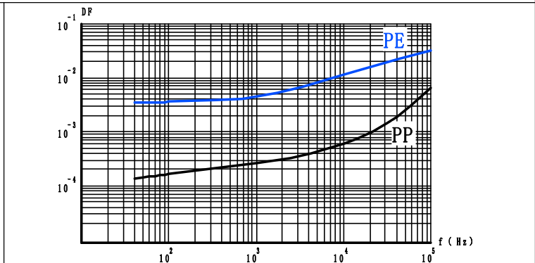
损耗角正切与频率的关系 Dissipation Factor vs. Frequency
