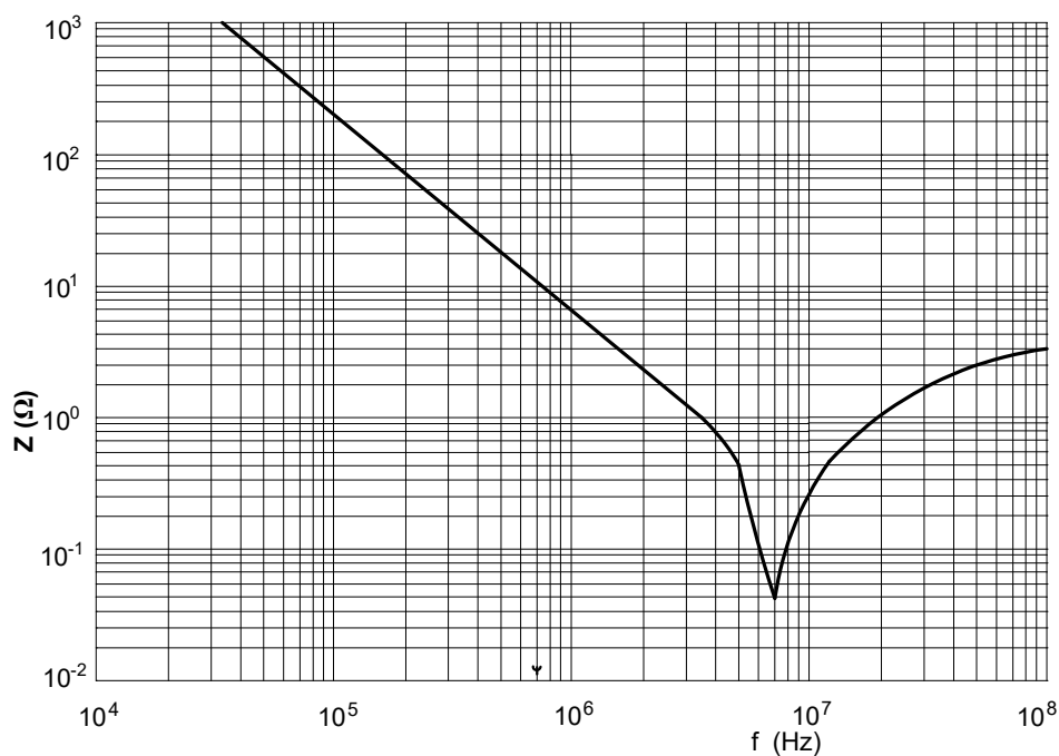
阻抗与频率 (典型值)
