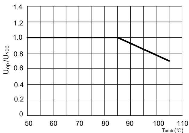
运行电压随温度变化曲线 (典型值)
