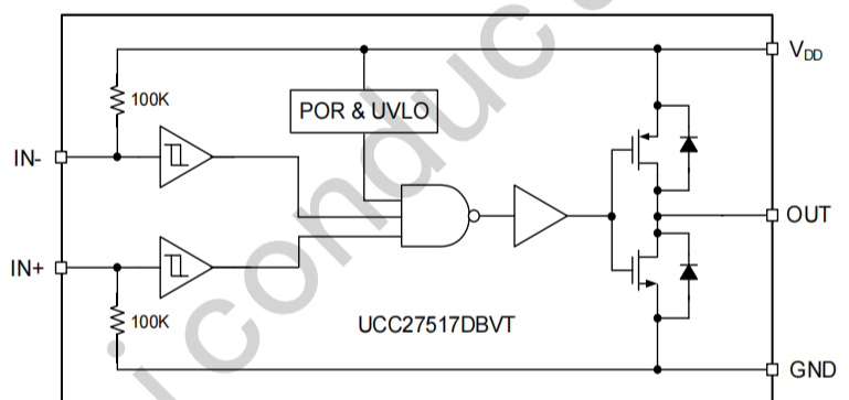
简化示意图
