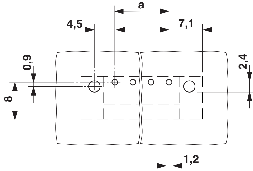
尺寸图
