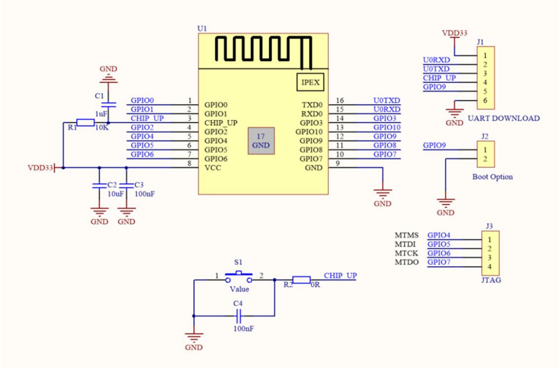
图 7 外围设计原理图
