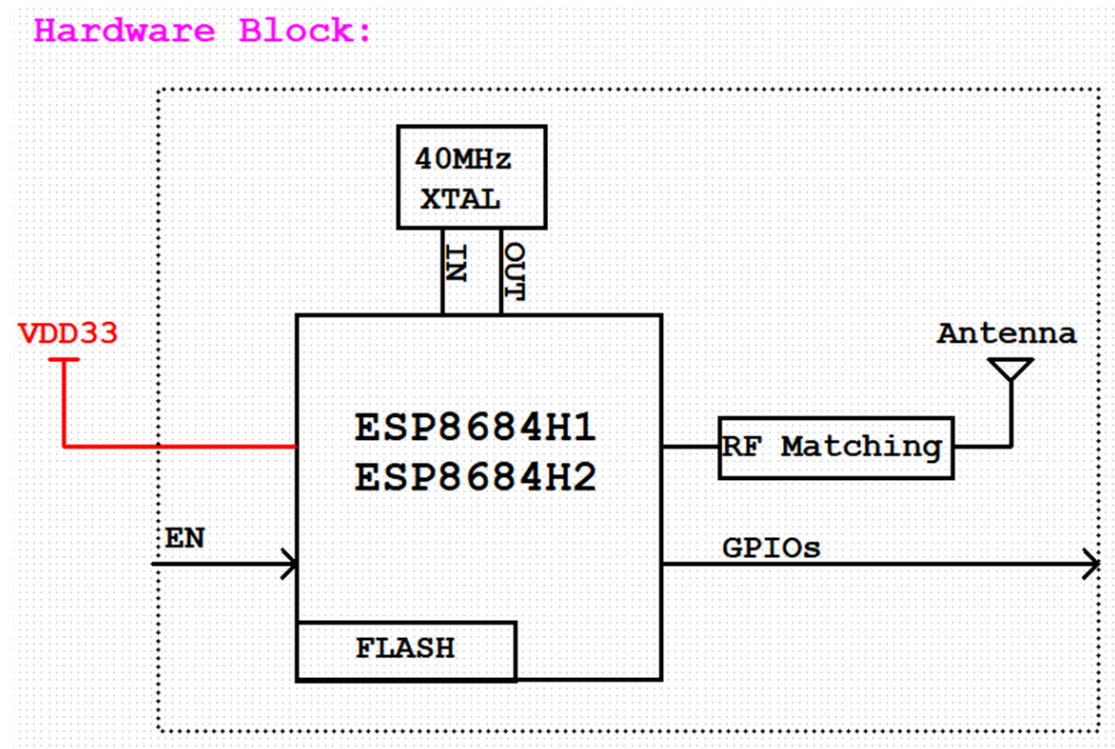
图 1 硬件框图
