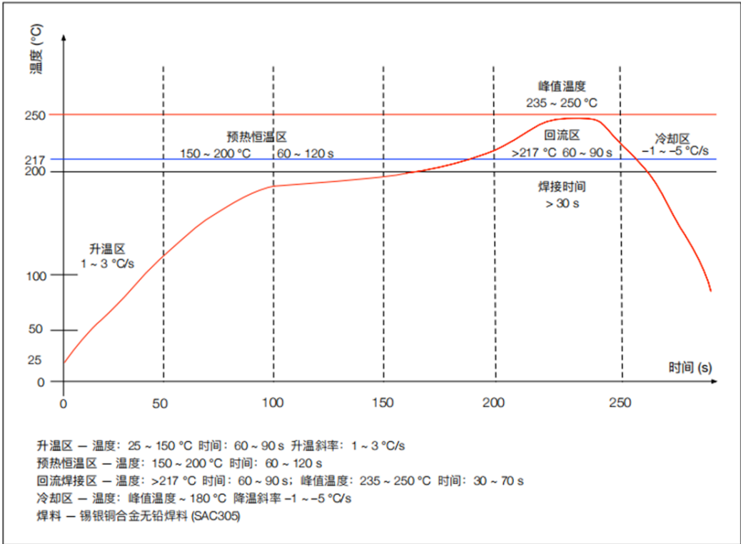
图 5 回流焊曲线
