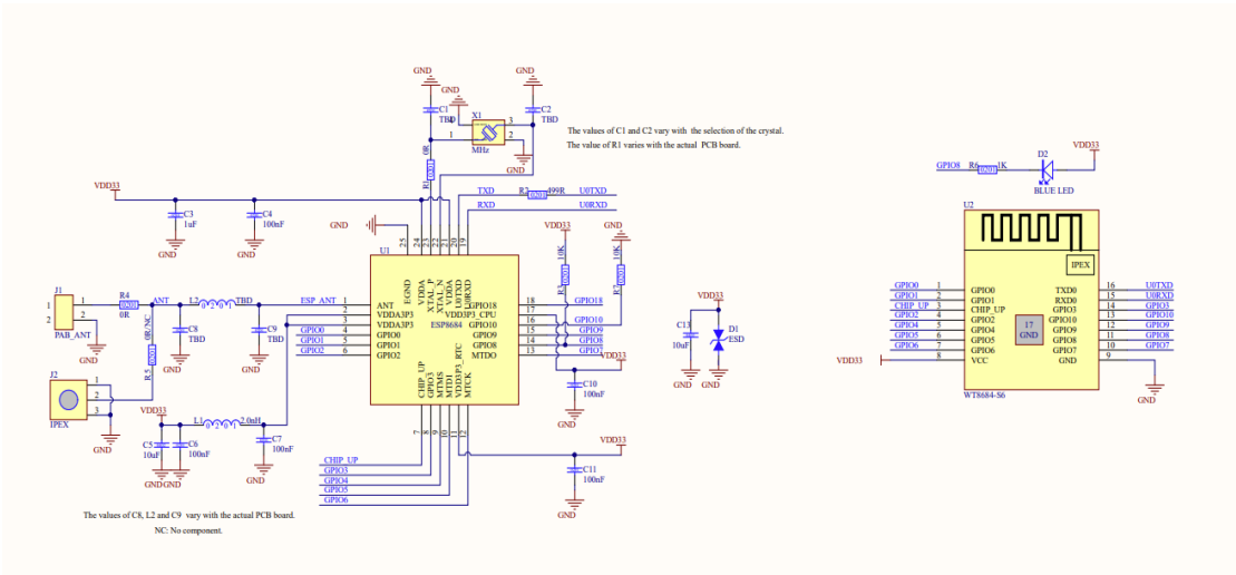
图 6 模组原理图
