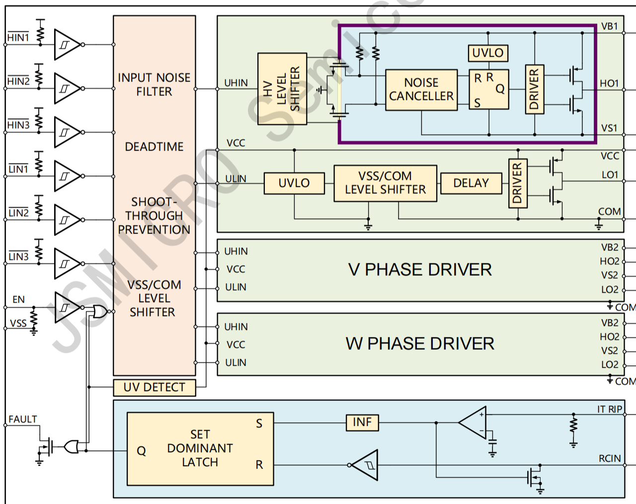
图7-1 TF2136M功能框图
