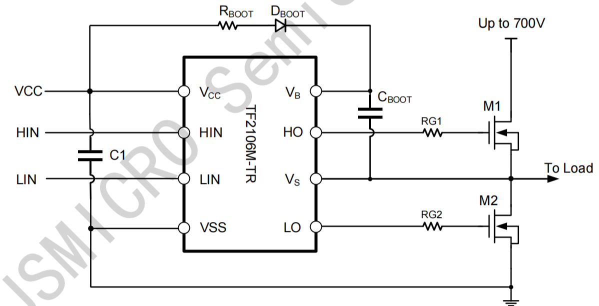
图 7-2 TF2106M典型应用电路图
