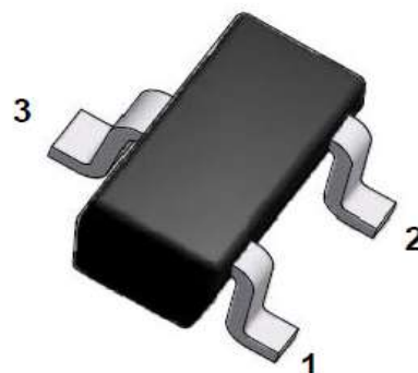
SOT-523 (SC-75A)
