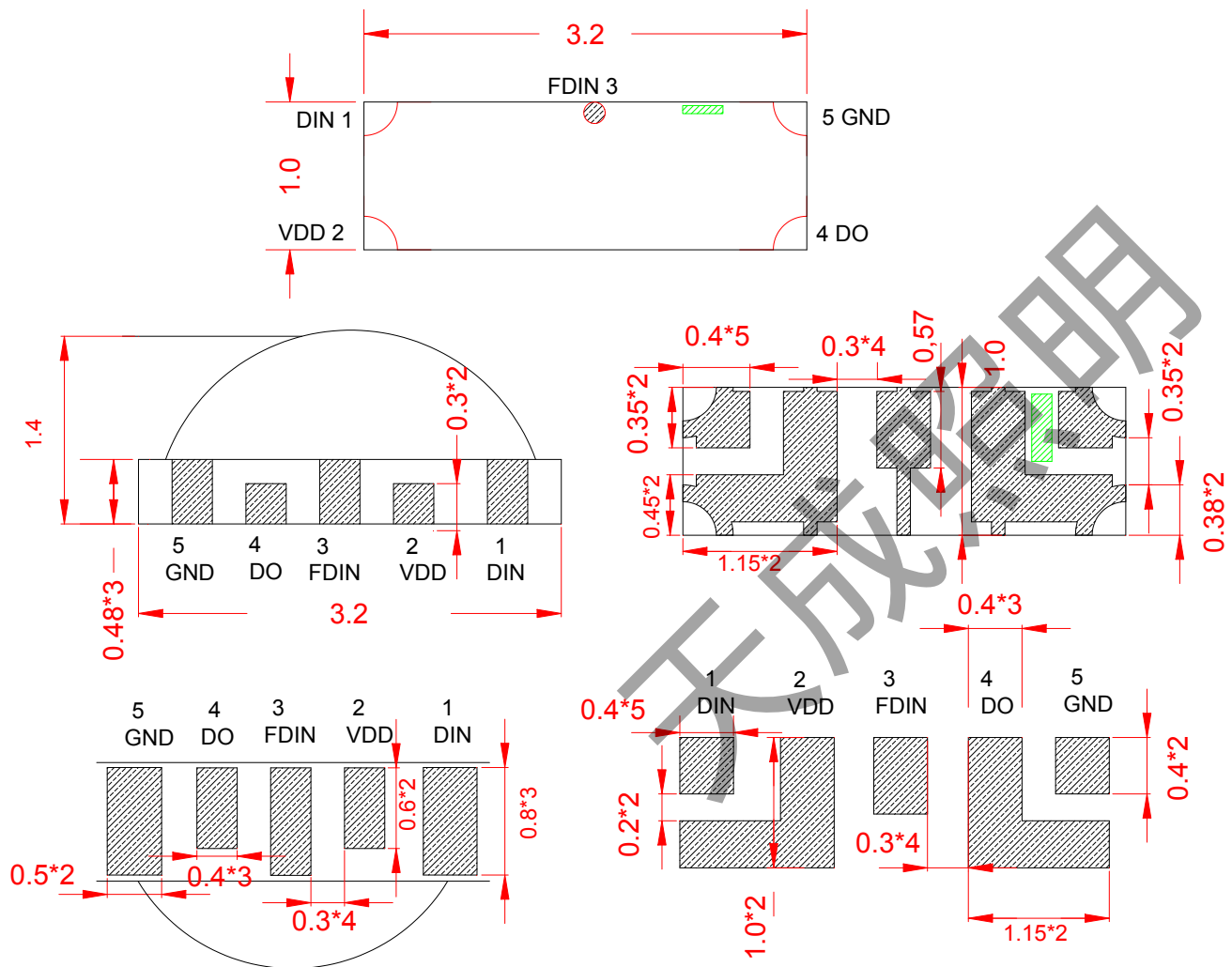
侧贴推荐焊盘尺寸
