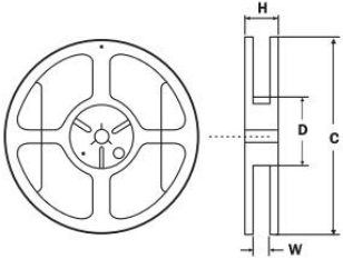
Reel Dimensions 卷盘规格
