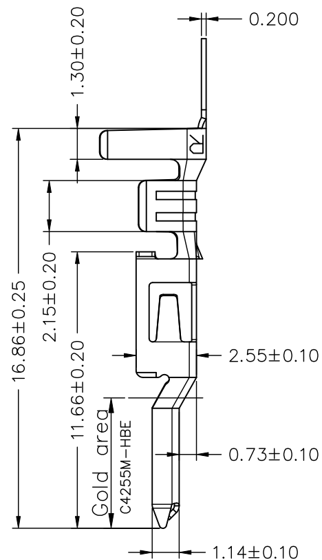
SEC: A-A
