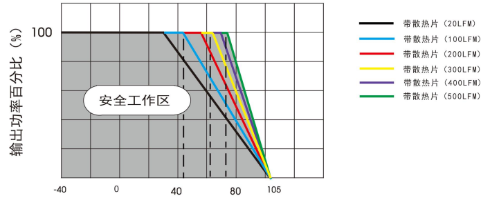
URF1D48HB-150WHR3 温度降额曲线(Vin=110V)
