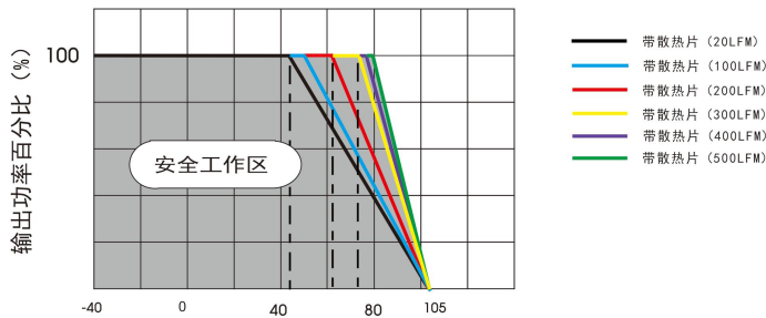
URF1D05HB-150WHR3 温度降额曲线(Vin=110V)
