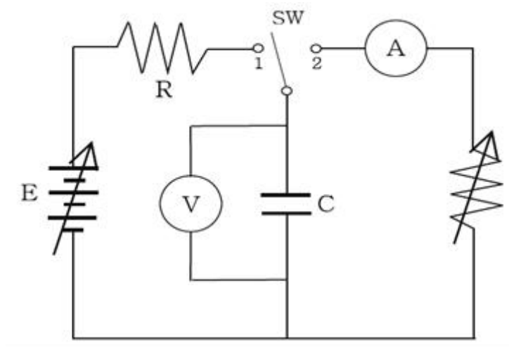
图1 容量测试电路图
