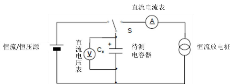
图1 恒流放电方法电路
