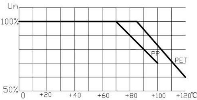
使用电压与温度的关系
