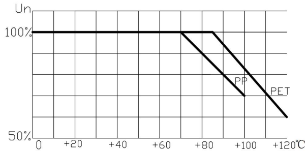
使用电压与温度的关系
