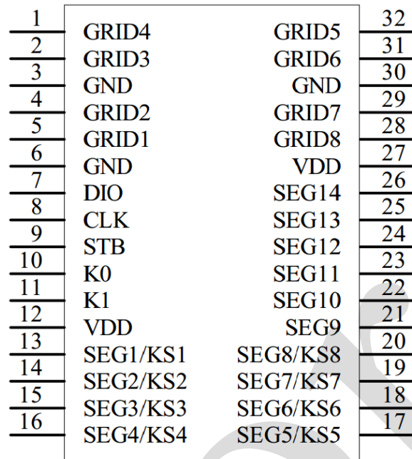
SOP32
