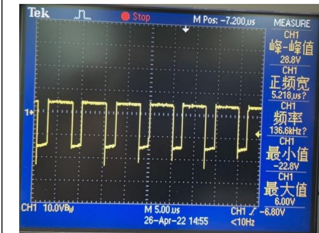
Rectifier diode
