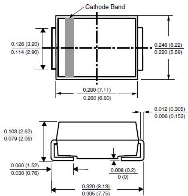
DO-214AB (SMC J-Bend)
