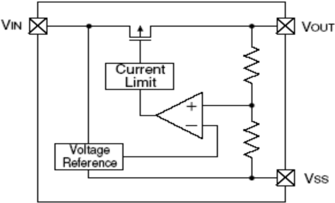
功能块框图
